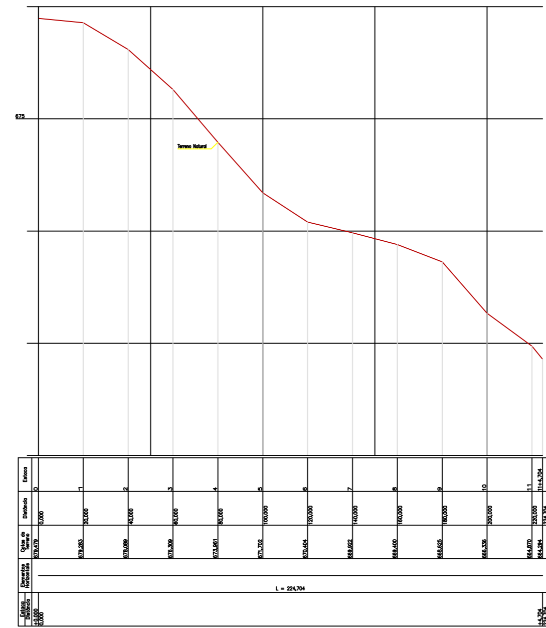
PERFIL LONGITUDINAL PARTE DA RUA JORGE LACERDA ESCALAS H 1:1000 - V 1:100
