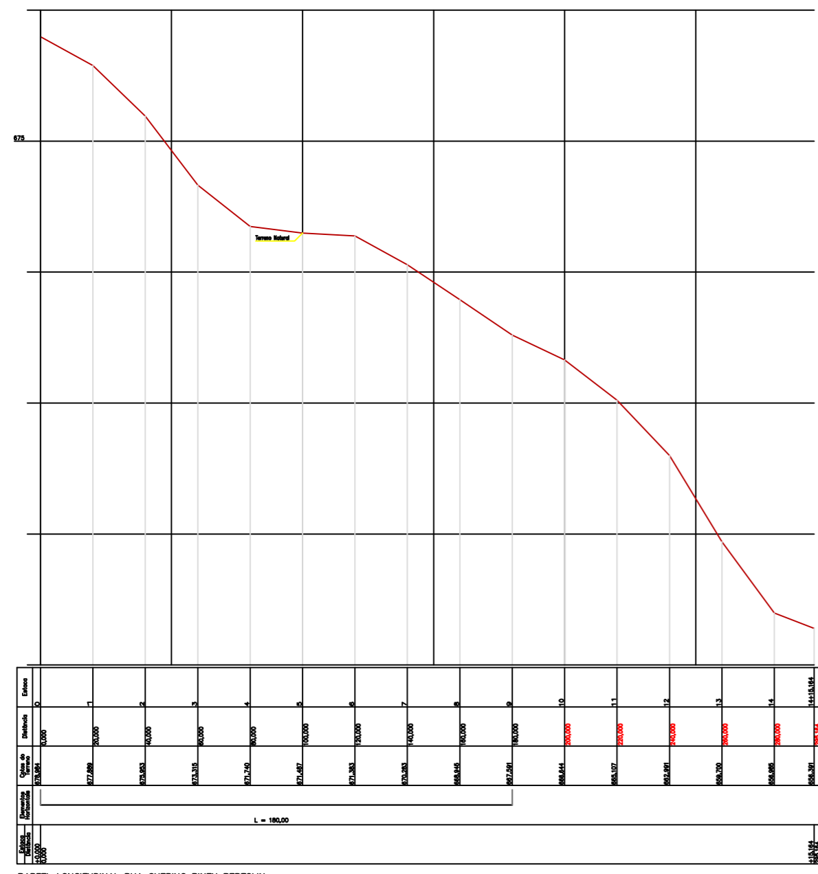
PARFEL LONGITUDINAL RUA GUERINO RINEU BERTOLIN ESCALAS H 1:1000 - V 1:100
