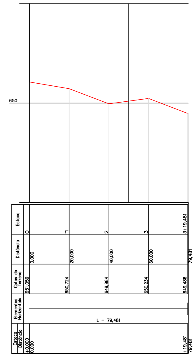
PERFIL LONGITUDINAL PARTE DA RUA JORGE LACERDA ESCALAS - H 1:1000 - V 1:100
