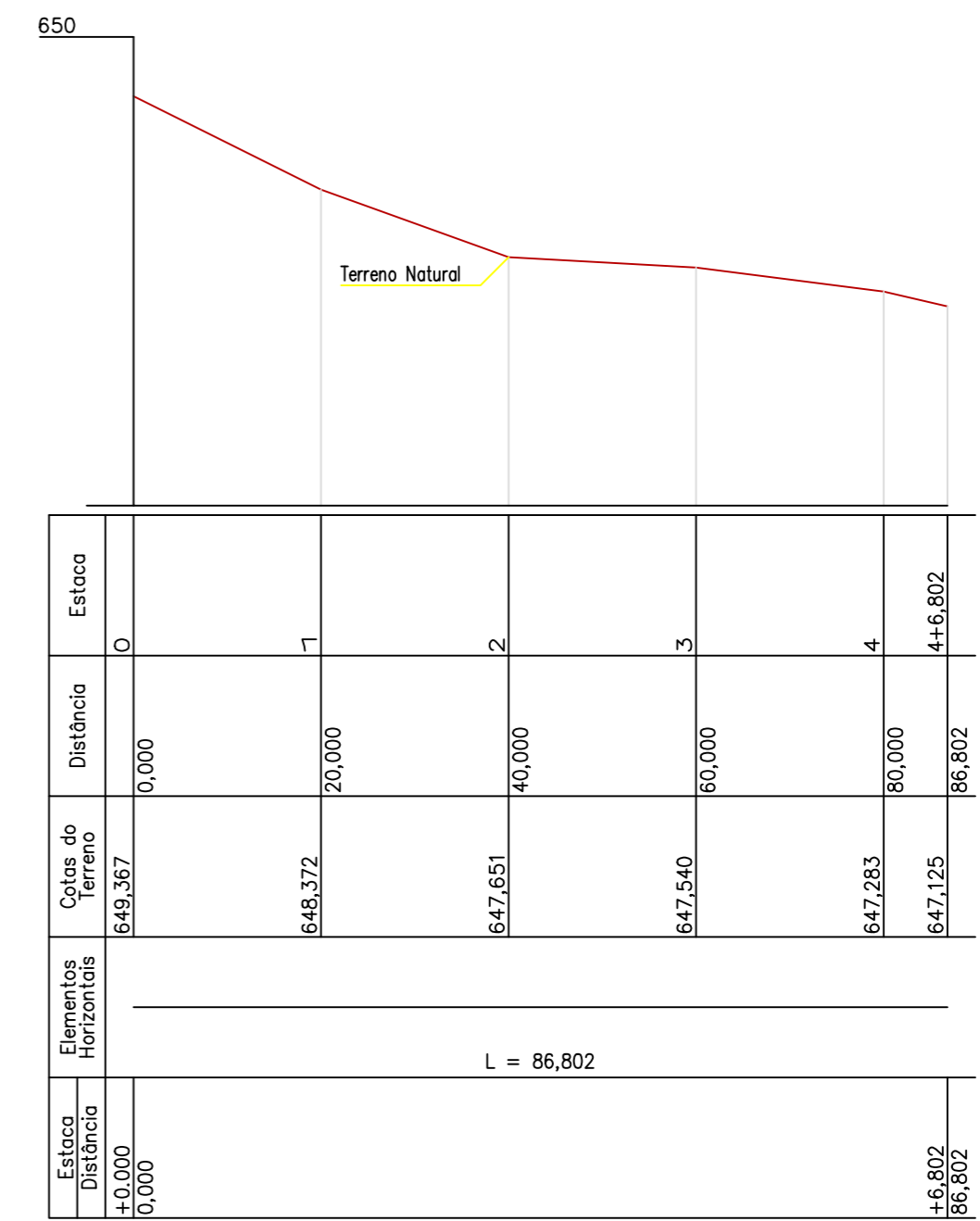
PERFIL LONGITUDINAL RUA FRANCISCO ROSA LIMA ESCALAS H 1:1000 – V 1:100
