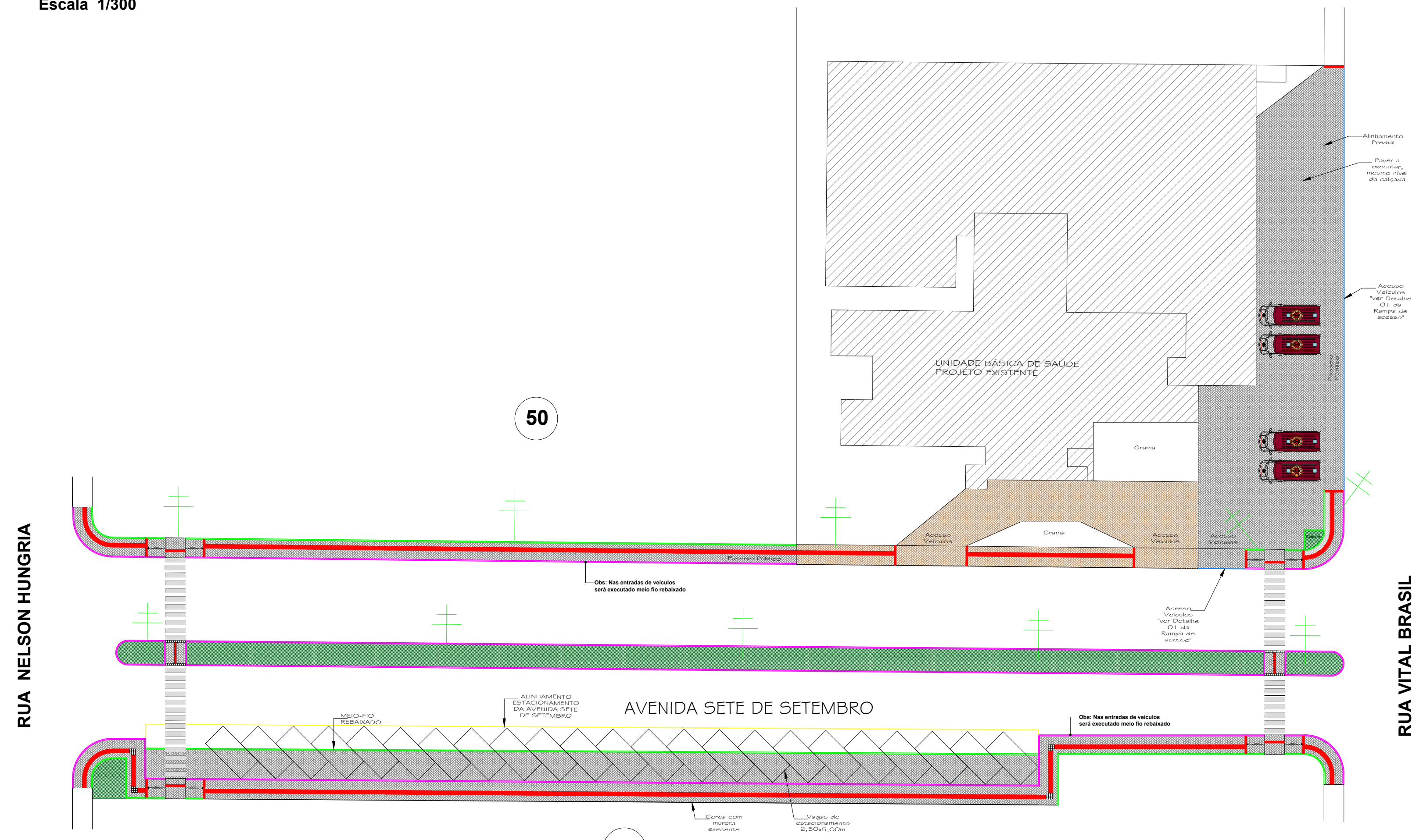
IMPLANTAÇÃO - PLANTA LAYOUT TRECHO 02 Escala 1/300
