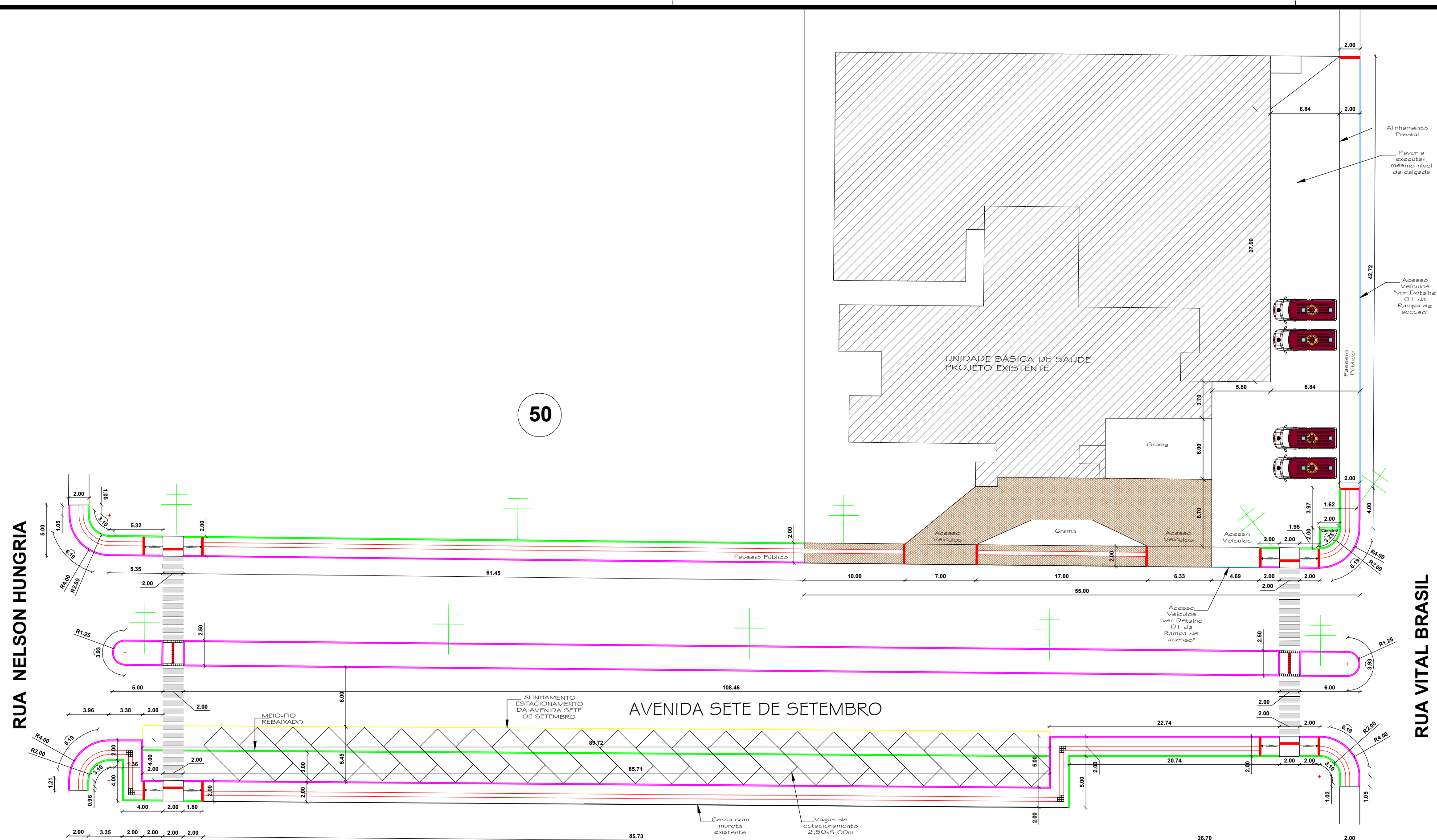
IMPLANTAÇÃO - PLANTA TÉCNICA TRECHO 02 Escala 1/300
