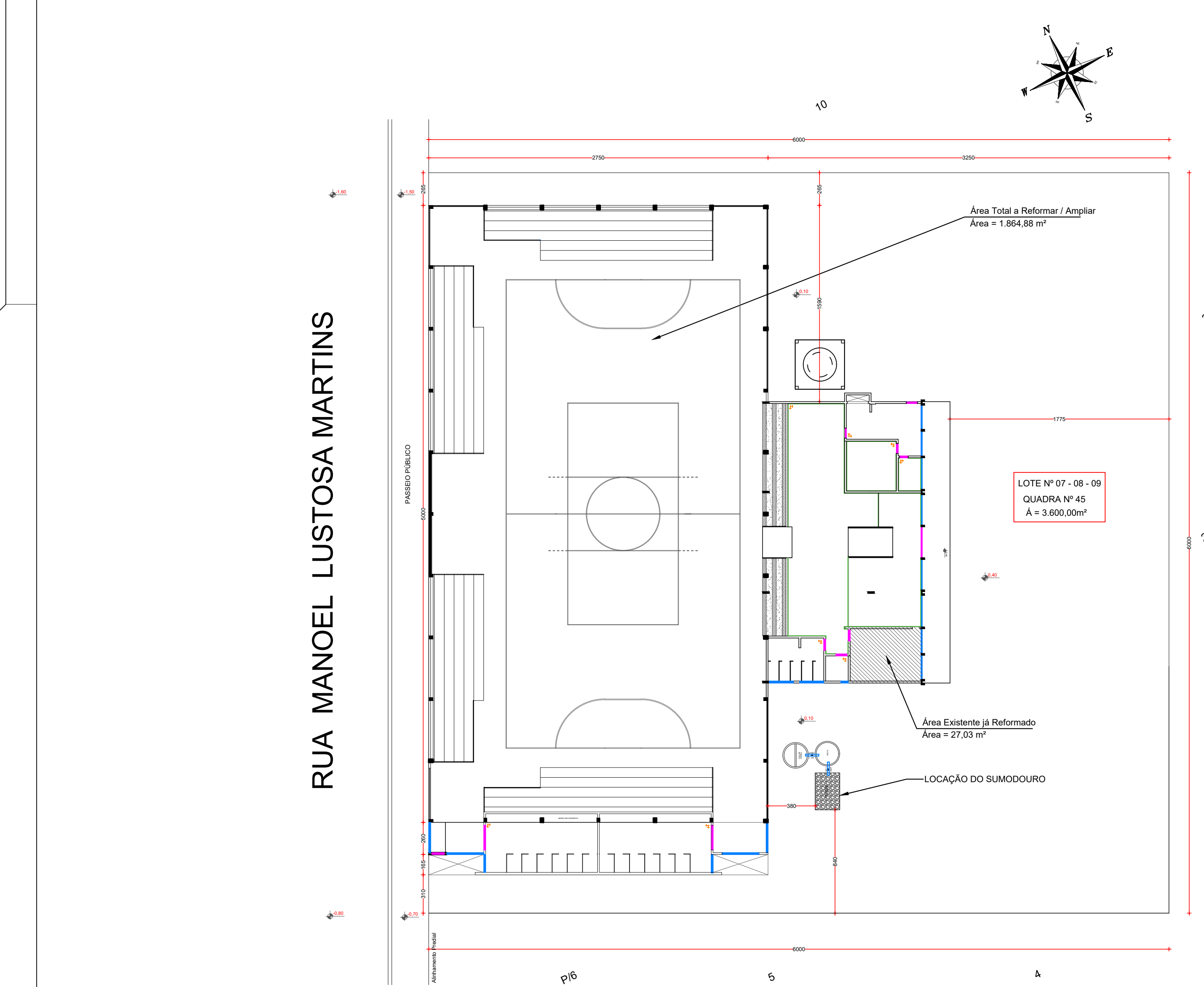
Implantação - Planta De Localização do Sumidouro Escala 1/200
