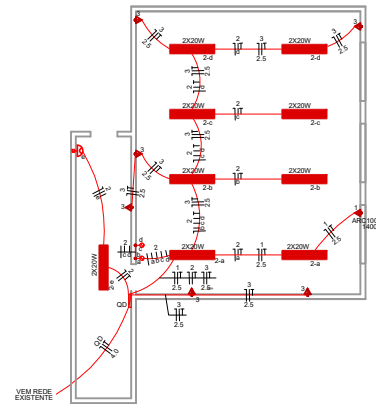
ELÉTRICO Esc.: 1/75
