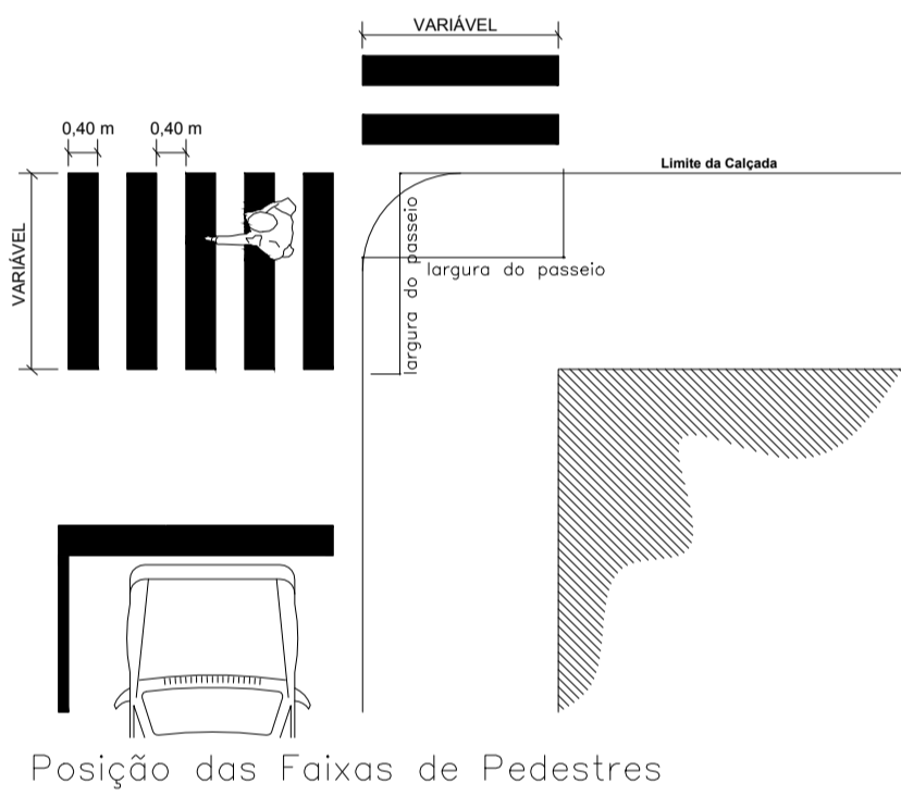
DETALHE PLACA R-19 SI ESCALA
