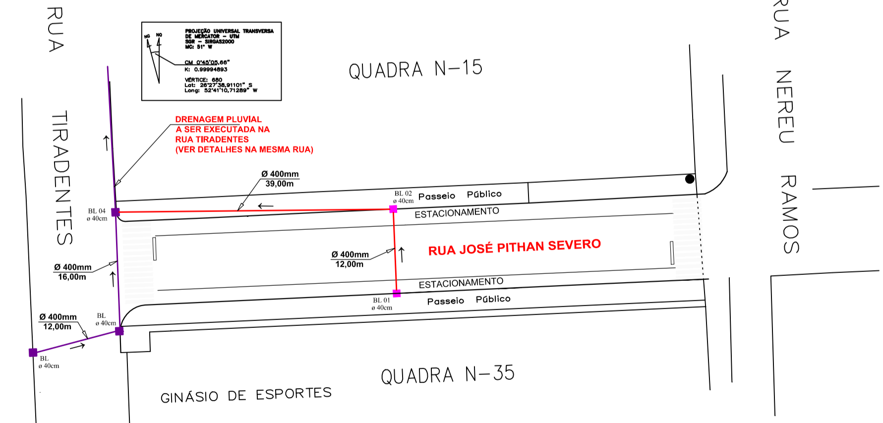
Drenagem Pluvial ESCALA 1 / 500
