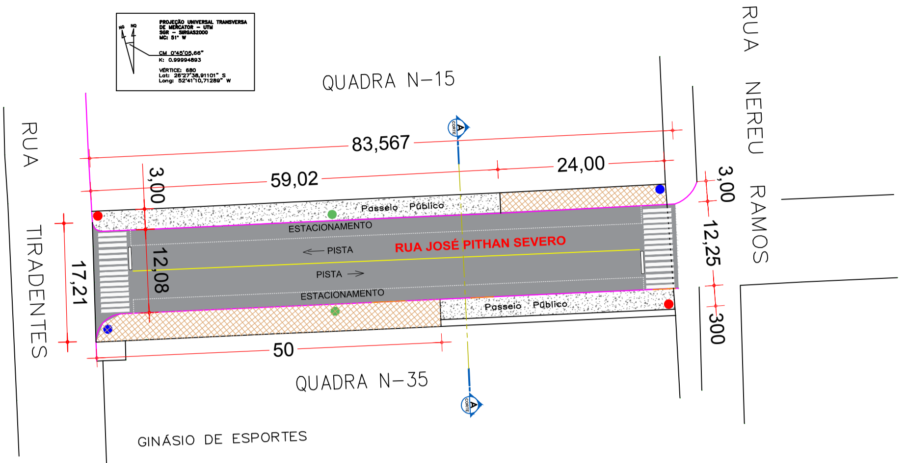
PAVIMENTAÇÃO ASFÁTICA P/ RUA JOSÉ PITHAN SEVERO ESCALA 1 / 500 ÁREA = 1.030,79m 2
