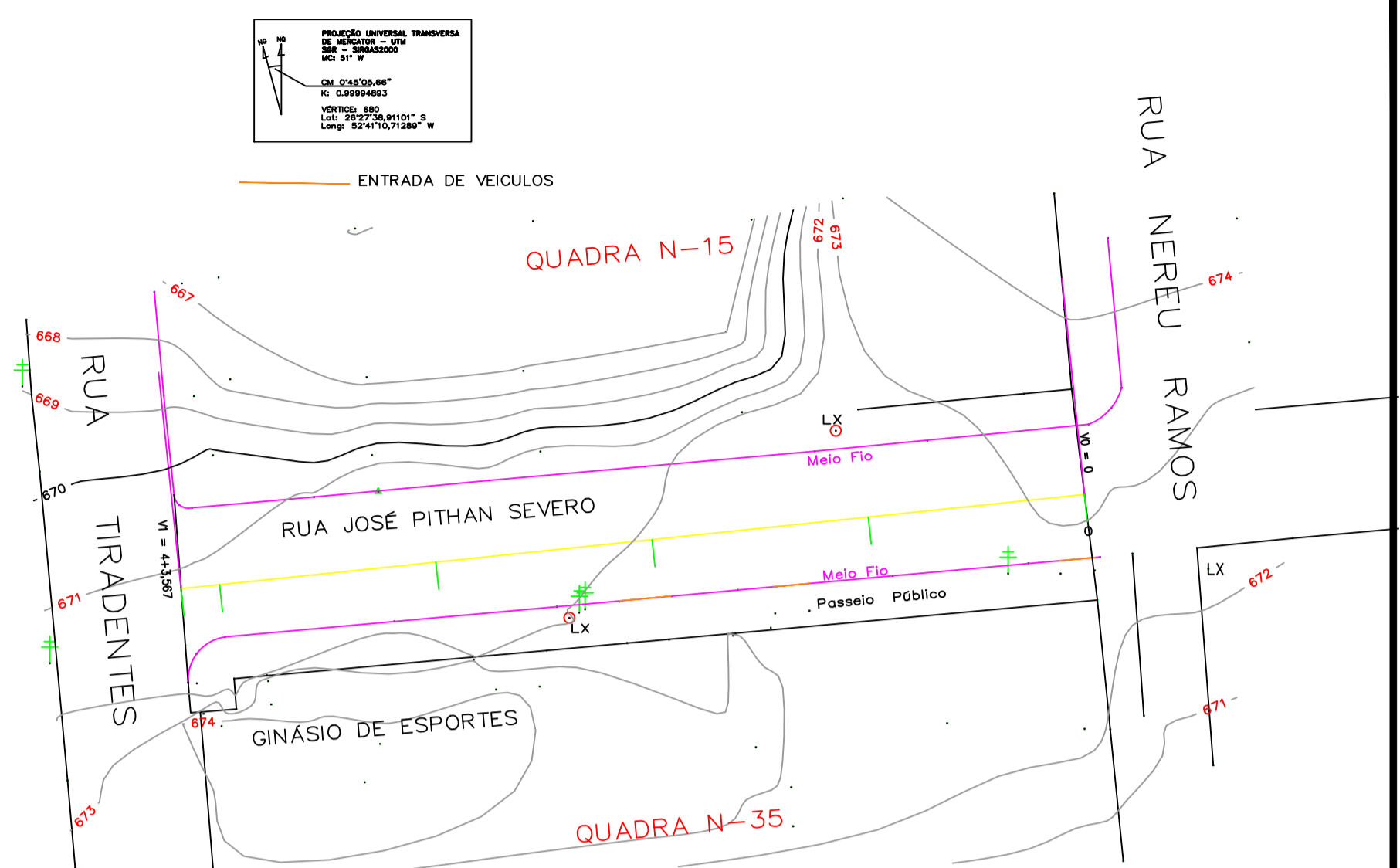
Planimétrico Escala 1/500
