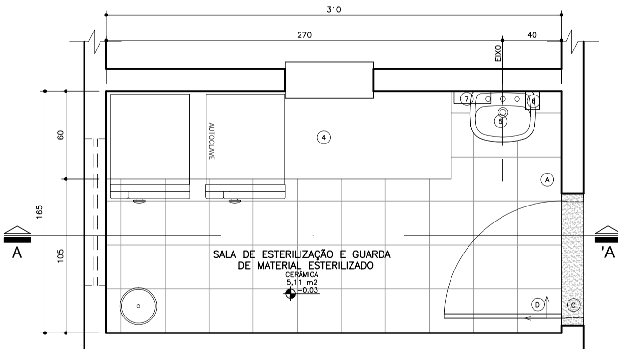
05 Planta Baixa Amb. 03 - ESTERILIZAÇÃO Esc.: 1:25
