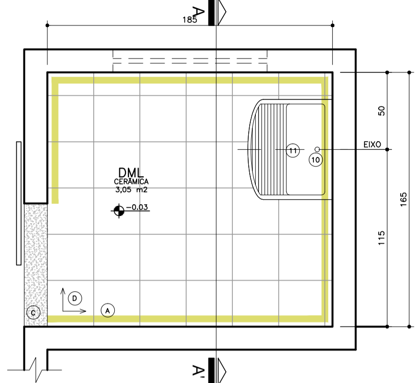
01 Planta Baixa Amb. 01 - DML Esc.: 1:25
