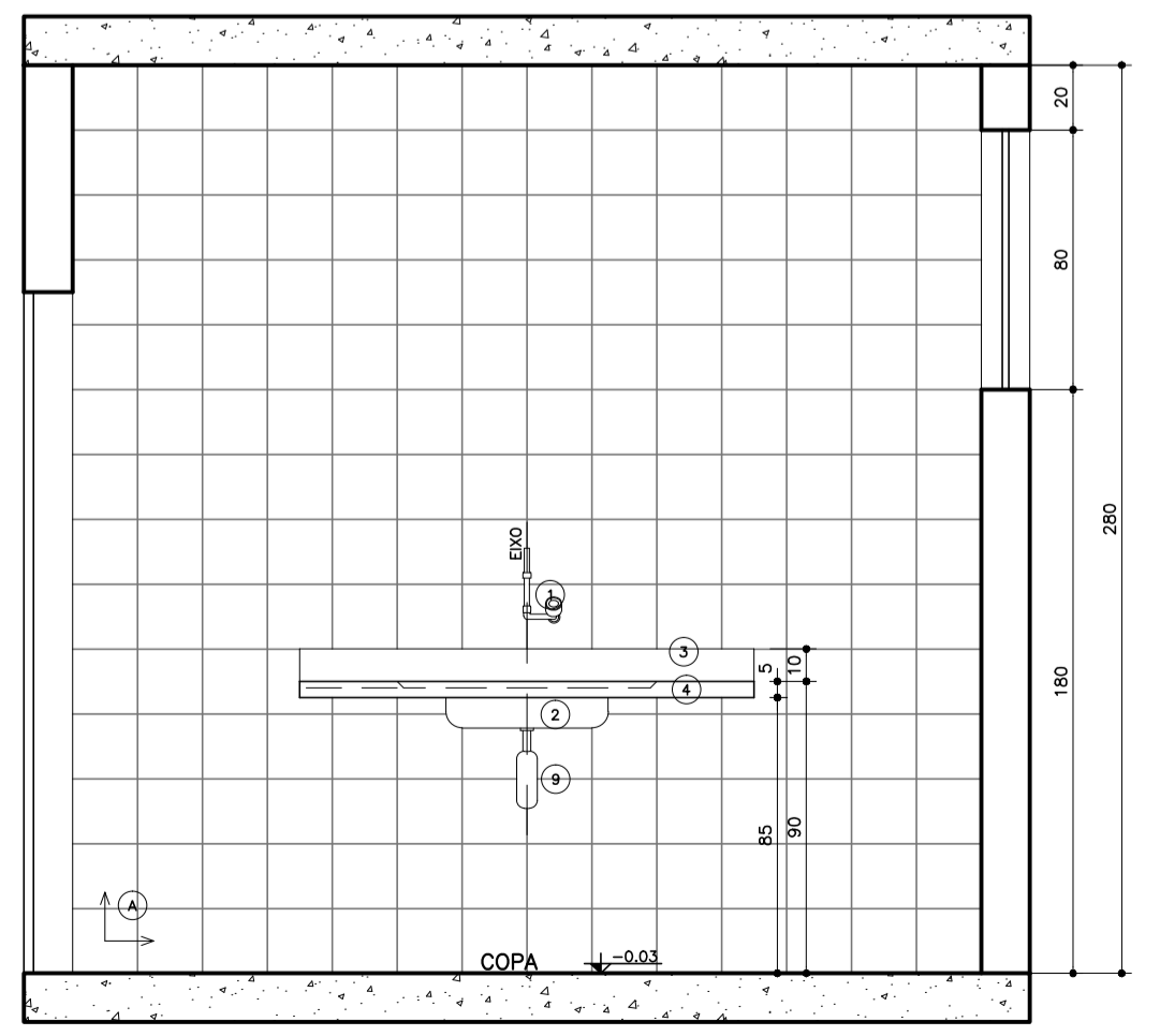
08 Seção AA' Amb. 04 - Copo Esc.: 1:25
