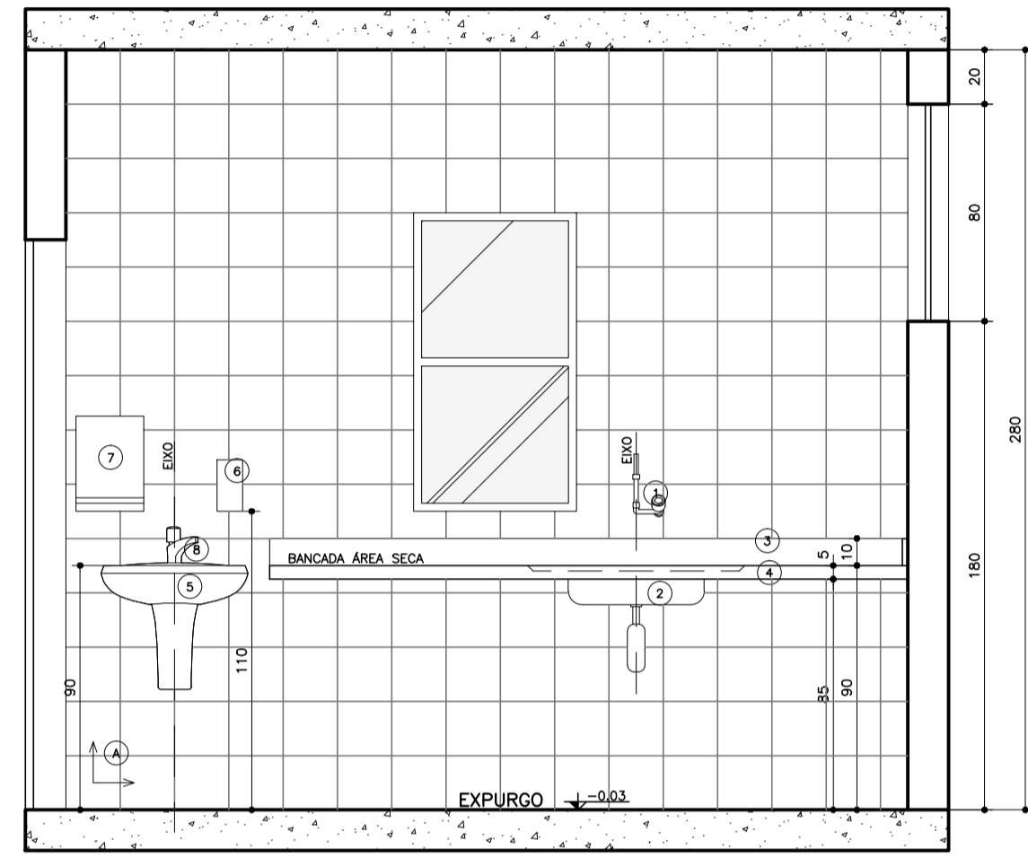
04 Seção AA' Amb. 02 - Expurgo Esc.: 1:25
