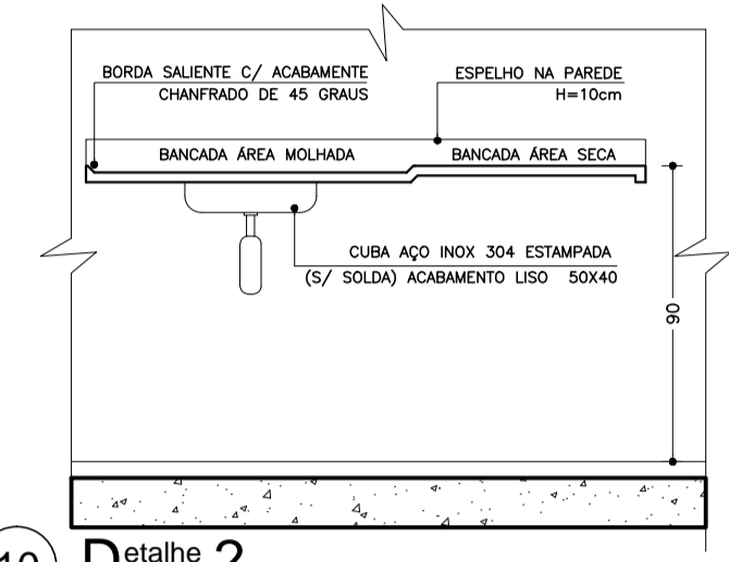
10 Detalhe 2 Esc.: 1:25
