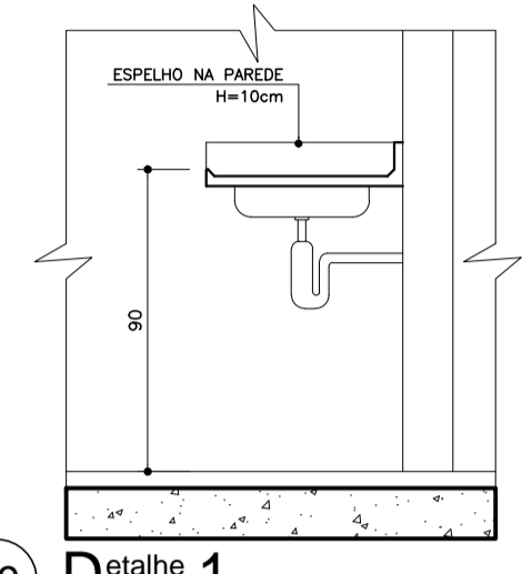
09 Detalhe 1 Esc.: 1:25
