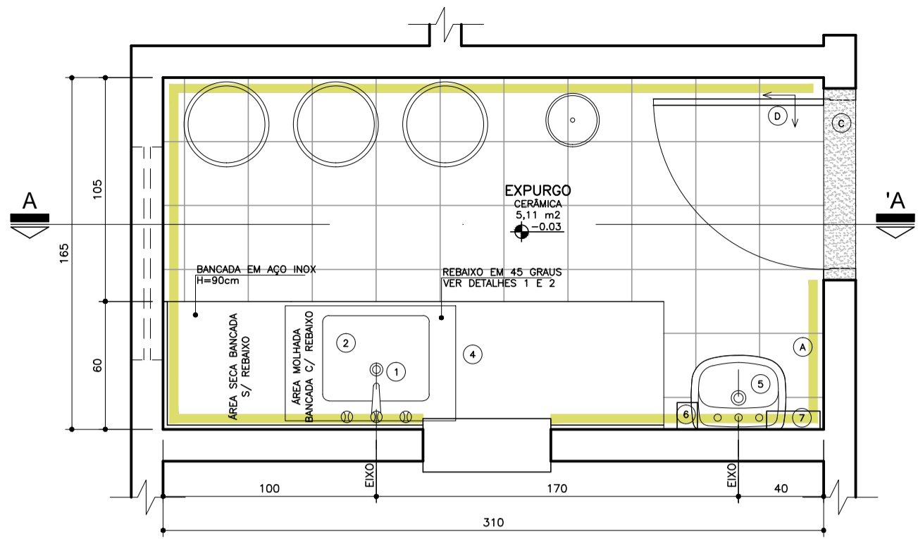
03 Planta Baixa Amb. 02 - EXPURGO Esc.: 1:25
